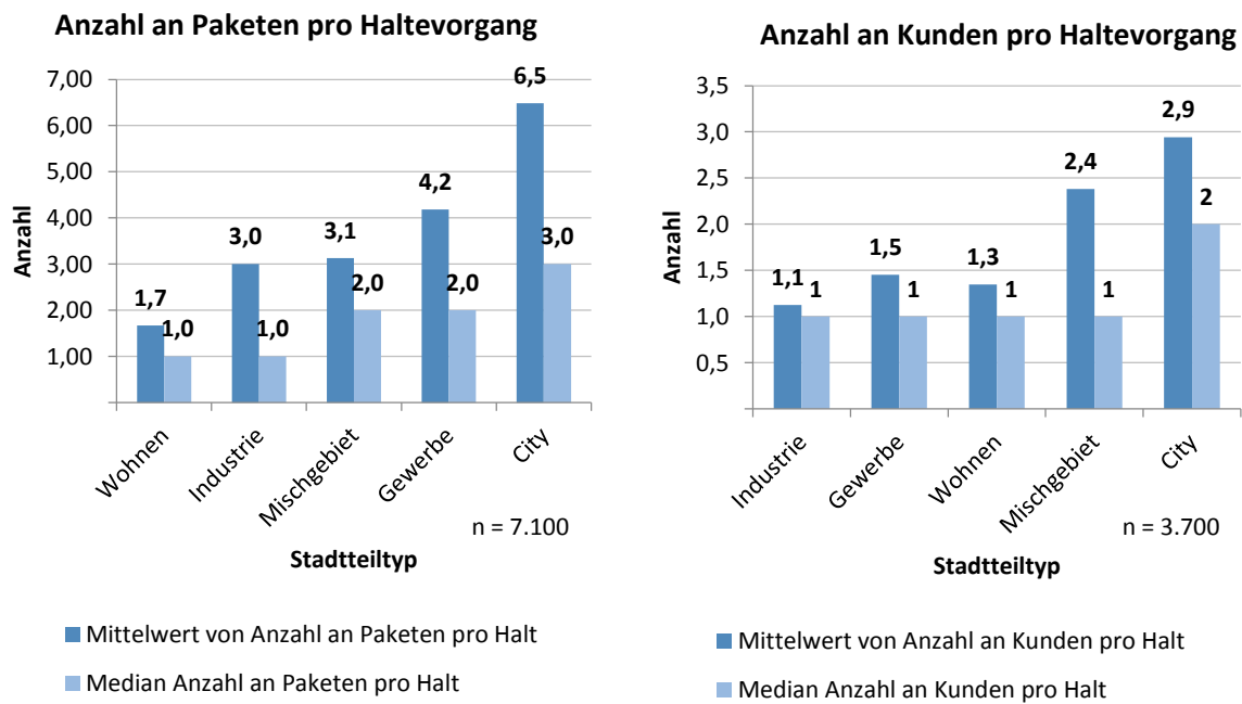
Abbildung 9: Anzahl an Paketen und Kunden pro Haltevorgang
