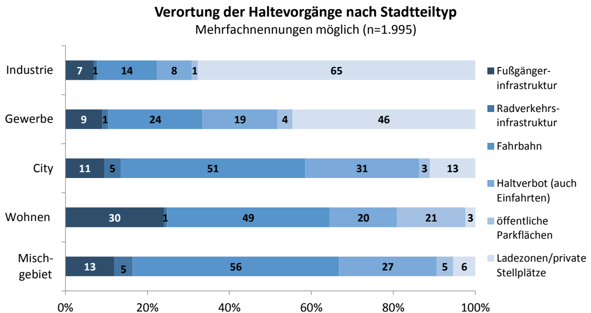
Abbildung 7: Prozentuale Anteile an Haltevorgänge nach Infrastruktur und Stadtteiltyp
