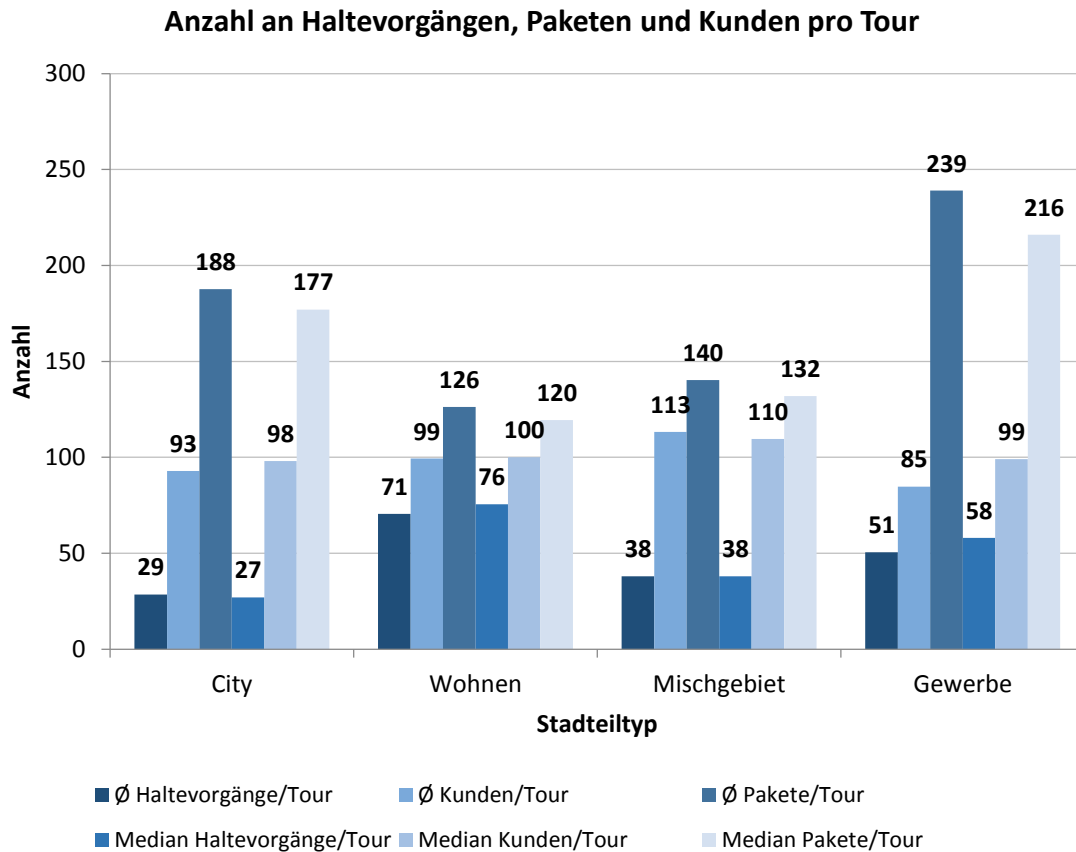
Abbildung 10: Anzahl an Haltevorgängen, Paketen und Kunden pro Tour und je Stadtteiltyp
